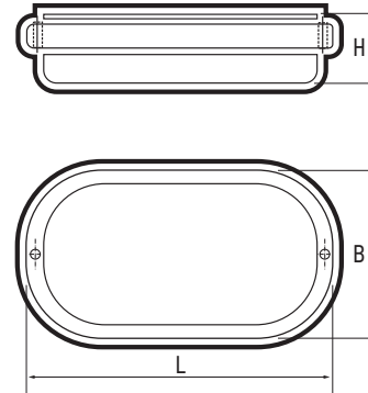
Рис. 2 Светильник PBH-PC7-0A
