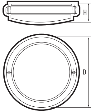
Рис. 1 Светильник PBH-PC7-RA
